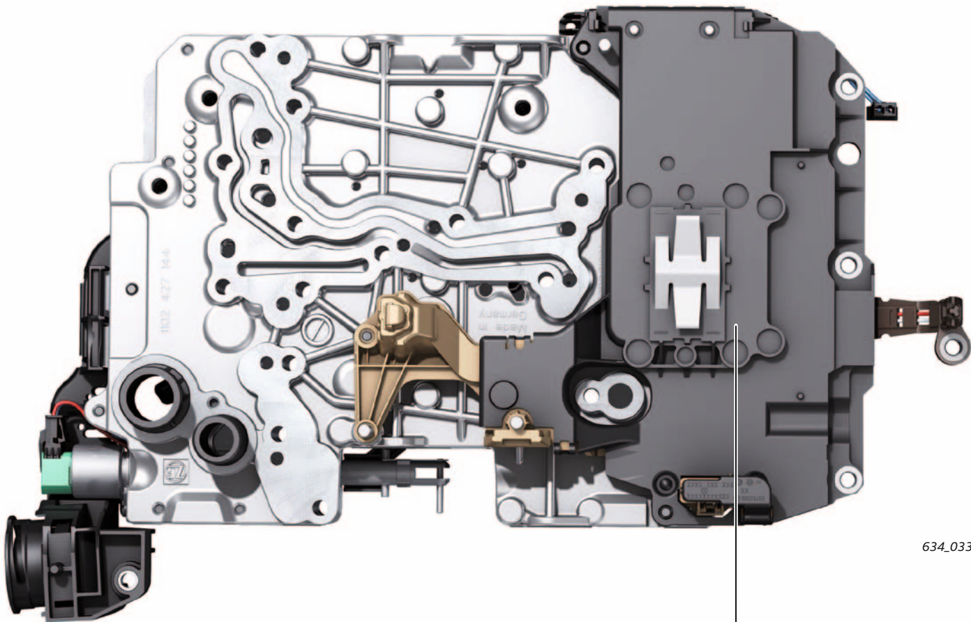
Steuergerät für automatisches Getriebe J217
