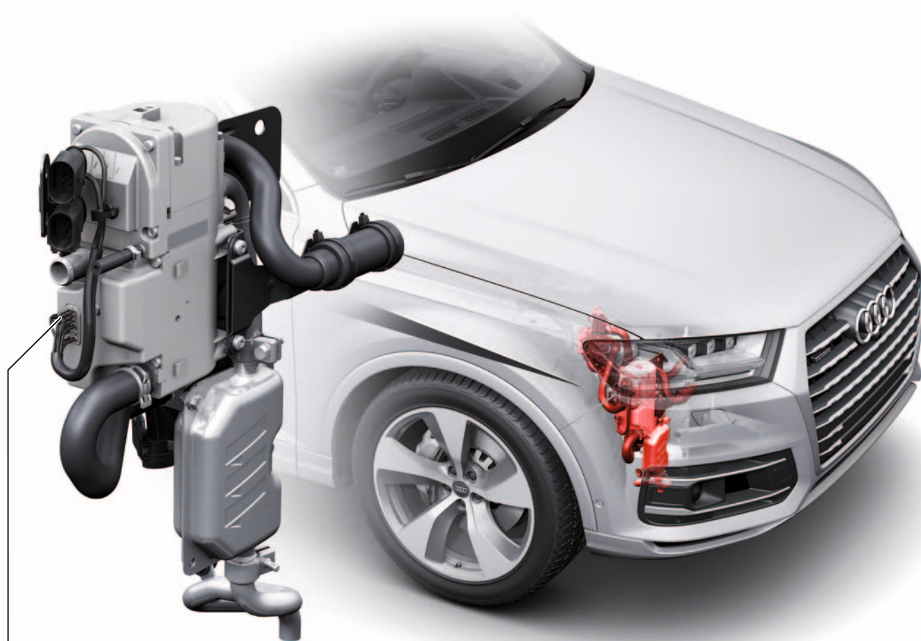
Steuergerät für Zusatzheizung J364
